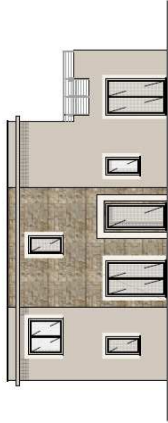
PROSPETTO EST
